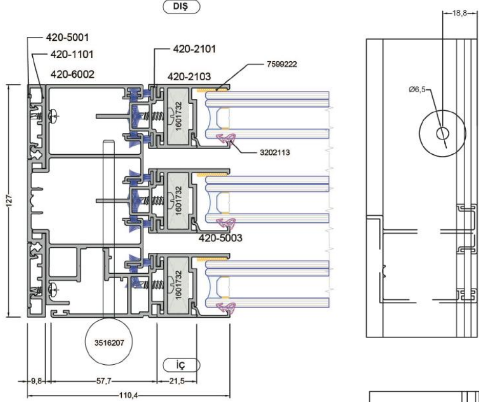
Yatay Kesit Açılır Pencere Güvenlik Pimi (Temizlik için)
