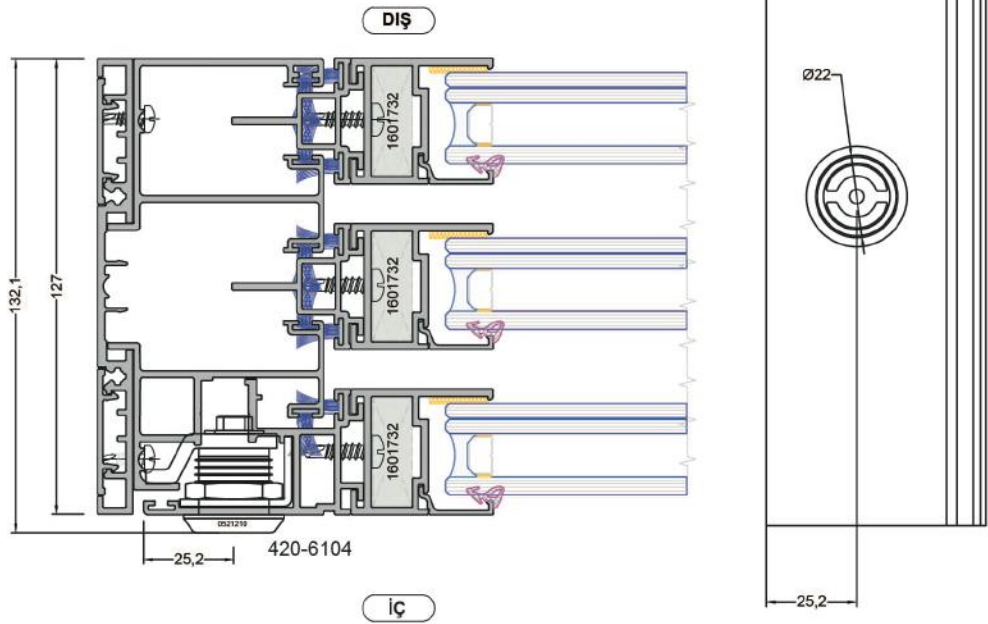
Yatay Kesit Açılır Pencere Kilit Mekanizması
