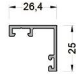
410-6009 (0,282 kg/mt ) GSAL100 MOTOR KUTU BİNİ PR.
