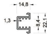
410-5001 ( 0,238 kg/mt ) TEK CAM ADAPTÖR PROFİLİ
