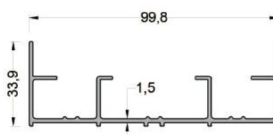
410-1102 ( 0,864 kg/mt ) GSAL100 KASA PROFİLİ
