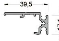
410-6002 (0,170 kg/mt ) GSAL100 KASA ADAPTÖR PRF.
