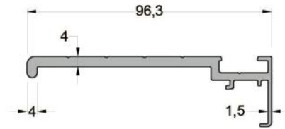
410-6006 (1,224 kg/mt ) GSAL100 KENET KAPAK 3'LÜ
