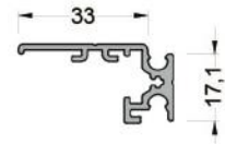
410-6009 (0,282 kg/mt ) GSAL100 MOTOR KUTU BİNİ PR.
