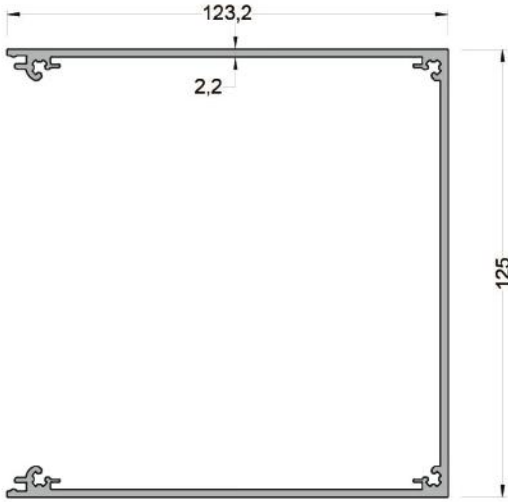
410-4004 ( 0,577 kg/mt ) GSAL100 MOTOR KUTU KAPAK PROFİLİ 125 mm
