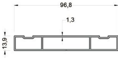
410-1101 ( 0,853 kg/mt ) GSAL100 KASA PROFİLİ
