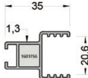
410-2102 ( 0,422 kg/mt ) GSAL100 KANAT PRF. 20 mm
