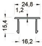
410-6003 (0,173 kg/mt ) GSAL100 RAY KAPAK PROFİLİ
