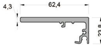
410-6005 (0,962 kg/mt ) GSAL100 KENET KAPAK 2'Lİ
