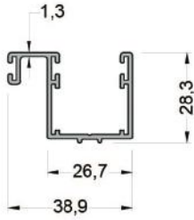
410-6001 (0,451 kg/mt ) GSAL100 SİSTEM RAY PROFİLİ
