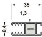
410-2101 ( 0,381 kg/mt ) GSAL100 TEKCAM KANAT PRF.
