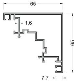
630-9101 (1,220 kg/mt) IP30C01 KÖŞE DÖNÜŞ
