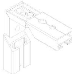
648-3102 ve 648-3103 KANAT İÇİN VİDALI 45° BAĞLANTI
