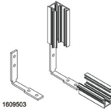
KASA - KASA BAĞLANTI 90°
