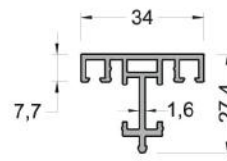
630-2101 (0,485 kg/mt) IP30M01 ORTA KAYIT
