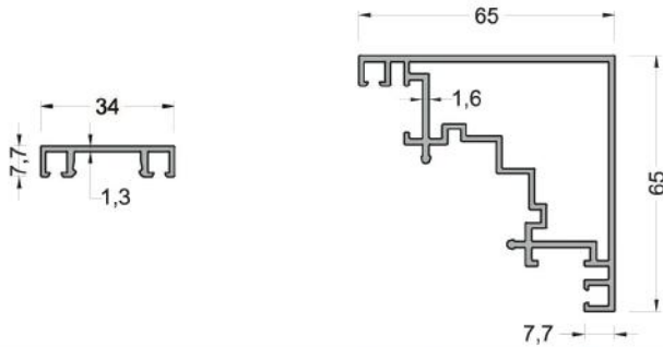
630-7201 (0,245 kg/mt) IP30P01 KAPAK
