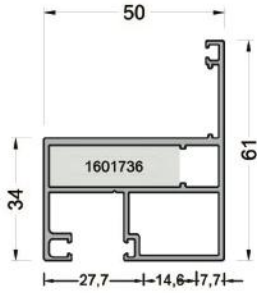
630-1101 (1,085 kg/mt) IP30F01 KASA PROFİLİ
