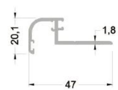
645-8102 (0,374 kg/mt ) IPA45A02 CAM KAPI ADAPTÖRÜ
