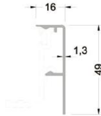
645-7101 (0,270 kg/mt ) IPA45P01 KAPAK PROFİLİ
