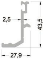
645-6201 (0,527 kg/mt ) IPA45P02 BASKI PROFİLİ
