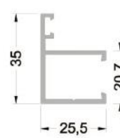
645-1202 (0,394 kg/mt ) IPA45F04 KASA PROFİLİ
