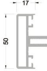
645-2101 (0,823 kg/mt ) IPA45M01 ORTA KAYIT PROFİLİ
