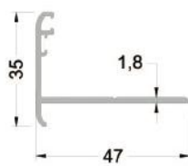
645-8101 (0,386 kg/mt ) IPA45A01 KANAT ADAPTÖR PR.
