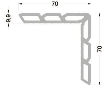
1099 (2,047 kg/mt ) L099 KÖŞE TAKOZU
