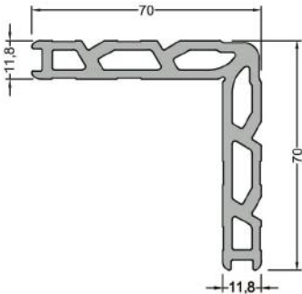
1118 (2,370 kg/mt) KÖŞE TAKOZU 11,8 mm 5022
