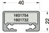
648-3102 (0,805 kg/mt) D48V02 KANAT PROFİLİ
