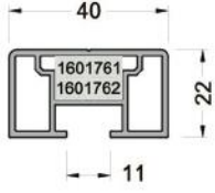
648-3108 (0,647 kg/mt) D48V08 KANAT PROFİLİ
