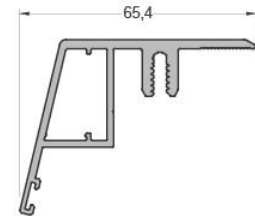
565-4201 ( 1,067 kg/mt ) SA65E01 KANAT KAPAK PROFİLİ
