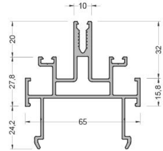
565-1103 ( 1,525 kg/mt ) SA65M03 DÜŞEY PROFİL
