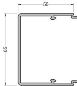
565-4101 ( 1,502 kg/mt ) SA65V01 KANAT PROFİLİ
