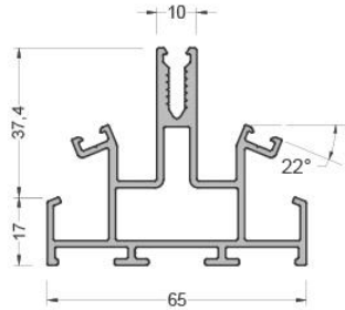
565-1102 ( 1,453 kg/mt ) SA65M02 DÜŞEY PROFİL
