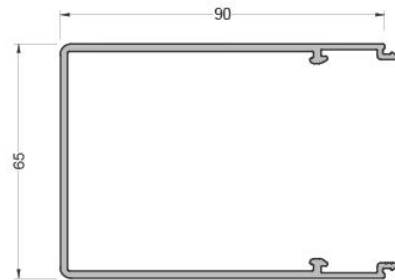
565-4201 ( 1,067 kg/mt ) SA65E01 KANAT KAPAK PROFİLİ
