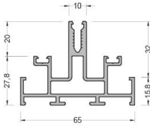
565-1101 ( 1,373 kg/mt ) SA65M01 DÜŞEY PROFİL
