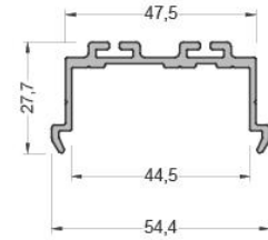
565-7101 ( 0,615 kg/mt ) SA65A01 BAĞLANTI PROFİLİ
