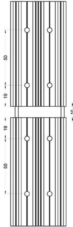
550-8101 ( 5,466 kg/mt ) W50D01 DILATASYON BAĞLANTI PROFİLİ
