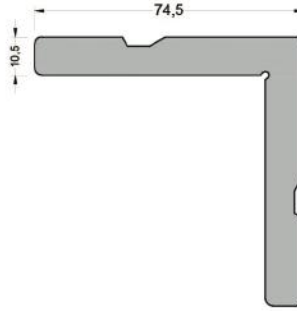
1105 ( 3,855 kg/mt ) L105 KÖŞE TAKOZU
