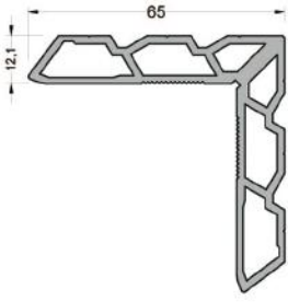
1121 ( 1,534 kg/mt ) L121 KÖŞE TAKOZU
