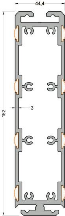
550-8101 ( 5,466 kg/mt ) W50D01 DILATASYON BAĞLANTI PROFİLİ
