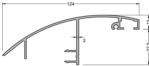
560-6003 (1,177 kg/mt) DERE KAPAK
