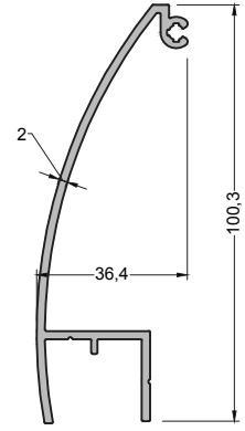
570-7104 (0,933 kg/mt) FRA80 A04 DERE ADAPTÖR PROFİLİ
