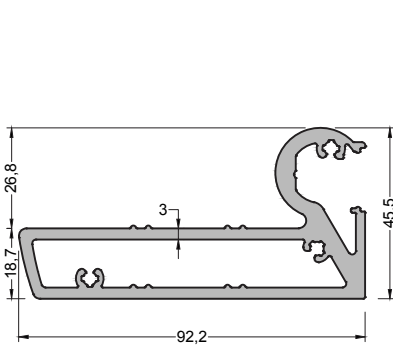
580-7106 (2,496 kg/mt) AÇILI ALT BAĞLANTI PROFİLİ
