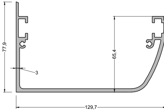
570-7103 (2,311 kg/mt) FRA80 A03 DERE PROFİLİ
