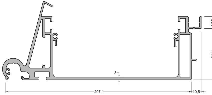
580-7105 (4,904 kg/mt) DERE PROFİLİ
