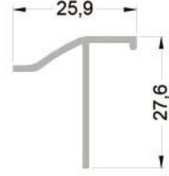
802-103 ( 0,195 kg/mt ) T03 T BİNİ PROFİLİ
