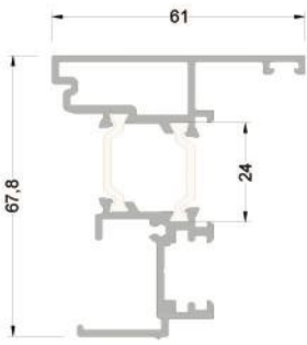
263-5101 ( 1,1400 kg/mt ) T63A01 ÇİFT KANAT ADPTR PR.
