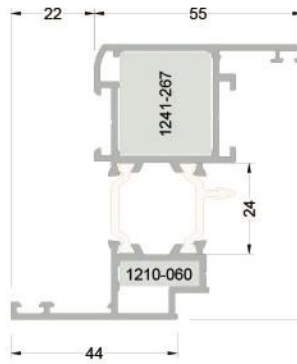
263-4401 ( 3,163 kg/mt ) T63K01 ETEK PROFİLİ
