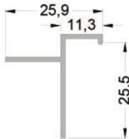
802-102 ( 0,188 kg/mt ) T02 T BİNİ PROFİLİ
