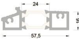
265-4101 ( 1,026 kg/mt ) T65K03 EŞİK PROFİLİ
