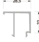
800-285 ( 0,300 kg/mt ) G285 CAM ÇİTASI
