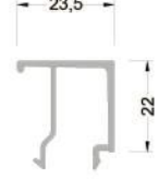
800-235 ( 0,280 kg/mt ) G235 CAM ÇİTASI
