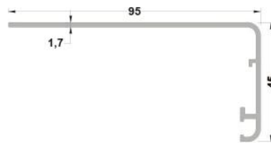
801-140 ( 0,605 kg/mt ) AW14 PERVAZ PROFİLİ
