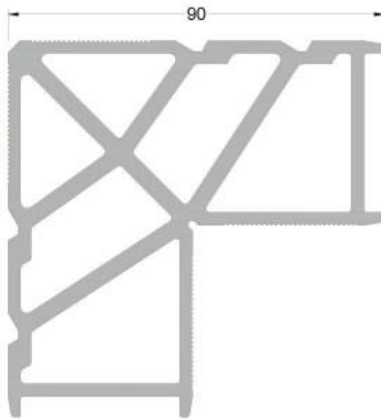
1441 ( 5,116 kg/mt ) L441 KÖŞE TAKOZU
