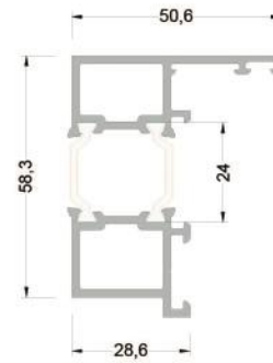
263-5103 ( 1,377 kg/mt ) T63A03 DIŞ AÇILIM ADPTR PR.
