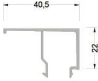
800-405 ( 0,340 kg/mt ) G405 CAM ÇİTASI
