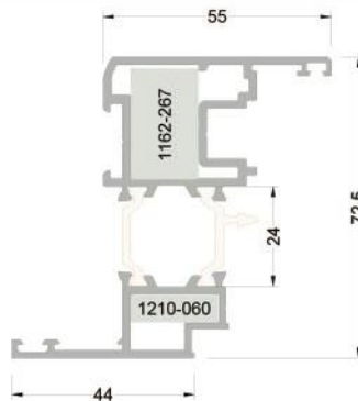
263-3608 ( 1,779 kg/mt ) T63V27 PVC KANAT PROFİLİ
