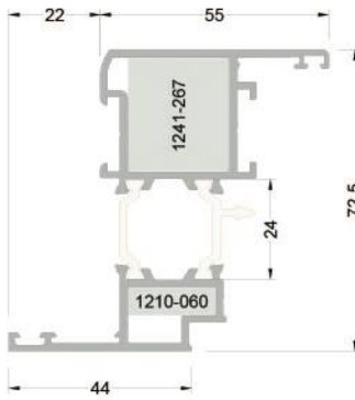
263-3204 ( 1,682 kg/mt ) T63V25 KANAT PROFİLİ
