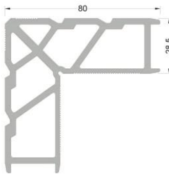
1162 ( 2,783 kg/mt ) L162 KÖŞE TAKOZU
