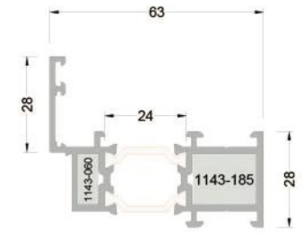
263-5105* ( 1,307 kg/mt ) T63A05 KANAT İÇİ KANAT ADP.
