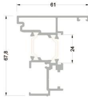
263-5102 ( 1,387 kg/mt ) T63A02 ÇİFT KANAT ADPTR PR.
