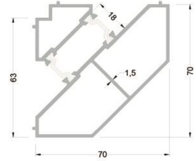
263-5106* ( 1,789 kg/mt ) T63A06 90° DÖNÜŞ ADAPTÖR PROFİLİ
