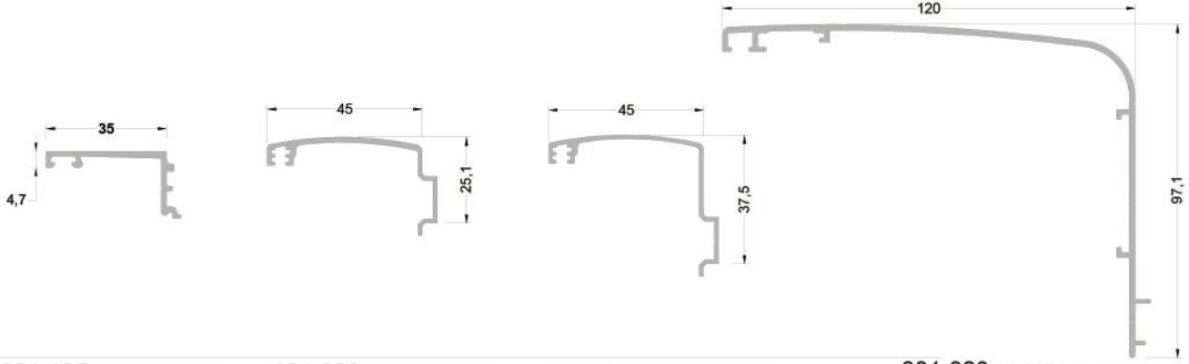
801-195 ( 0,293 kg/mt ) AW01 PERVAZ PROFİLİ
