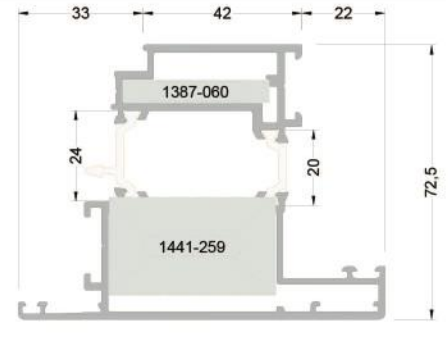
263-3403 ( 2,323 kg/mt ) T63V11 DIŞ AÇILIM KAPI KANAT PROFİLİ
