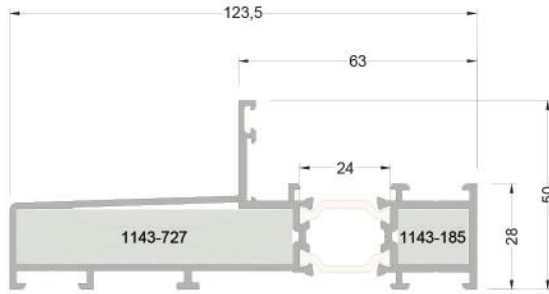
320-1403 ( 1,970 kg/mt ) ST120F08 SABİT GEÇİŞ KASA PROFİLİ
