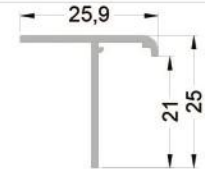
802-101 ( 0,185 kg/mt ) T01 T BİNİ PROFİLİ
