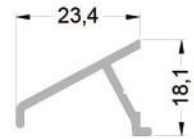
803-101 ( 0,186 kg/mt ) P01 DAMLALIK PROFİLİ
