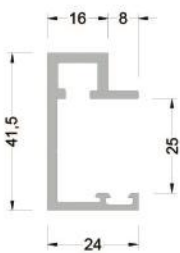
AS-8255 ( 0,681 kg/mt ) CAM KORKULUK DİKME PR.
