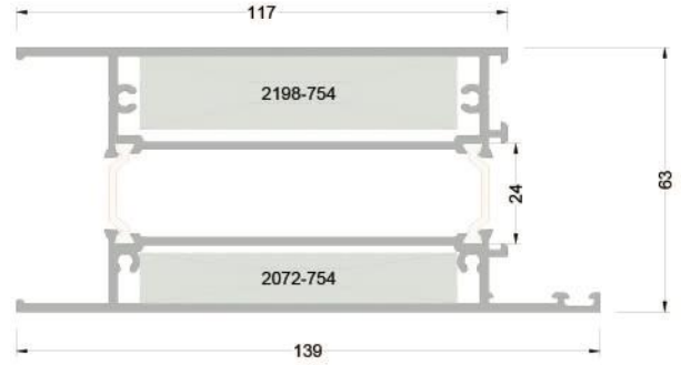
263-4401 ( 3,163 kg/mt ) T63K01 ETEK PROFİLİ
