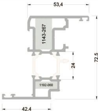
263-3603 ( 1,764 kg/mt ) T63V17 PVC KANAT PROFİLİ
