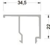
800-345 ( 0,320 kg/mt ) G345 CAM ÇİTASI
