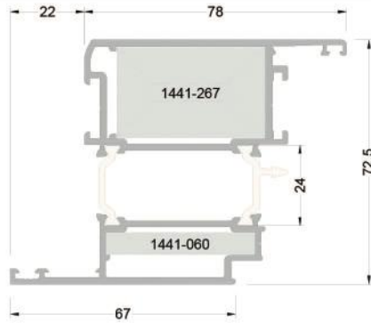
263-3401 ( 2,223 kg/mt ) T63V09 KAPI KANAT PROFİLİ
