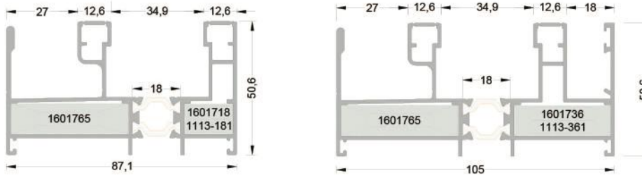
310-1207 ( 1,742kg/mt ) SLAT64 F12 SİNEKLİK RAYLI KASA PROFİLİ
