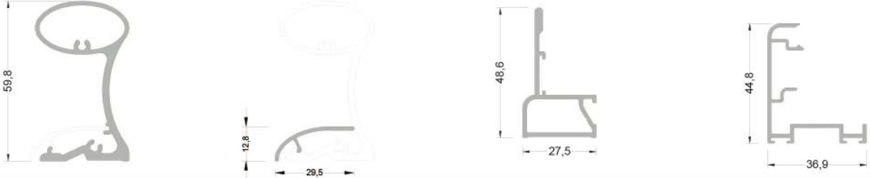
380-6003 ( 0,960 kg/mt ) SLA-A02 TAKVİYE PROFİLİ
