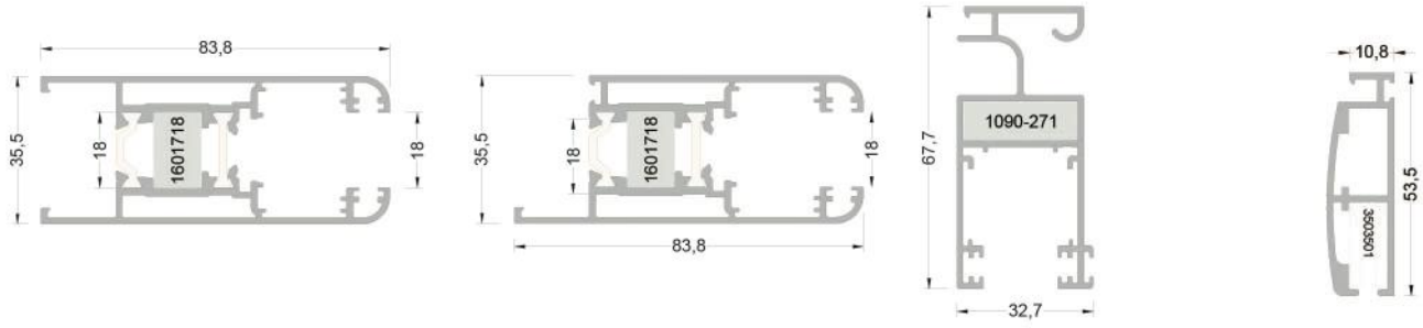
310-2101 ( 1,578 kg/mt ) SLT64V01 KANAT PROFİLİ
