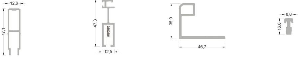
380-6005 ( 0,463kg/mt ) SLA-A04 4LÜ KANAT ADAPTÖRÜ
