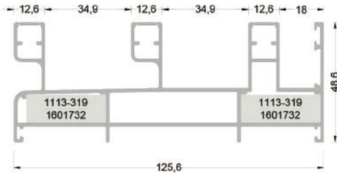
300-1302 ( 2,030 kg/mt ) SL60F05 3'LÜ KASA PROFİLİ
