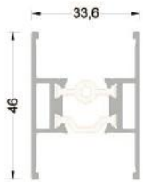
300-1302 ( 2,030 kg/mt ) SL60F05 3'LÜ KASA PROFİLİ
