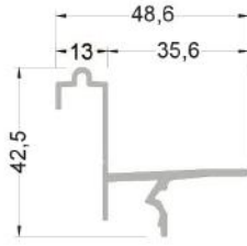
360-4002* ( 0,444 kg/mt ) SİNEKLİK RAY PROFİLİ
