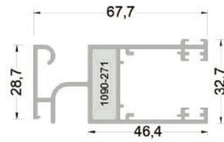
380-4006 ( 1,003 kg/mt ) SLA-S01 SİNEKLİK KANAT PR.
