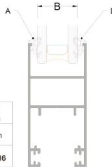
801-070 ( 0,522 kg/mt ) PERVAZ PROFİLİ
