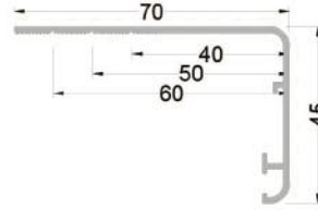
801-070 ( 0,522 kg/mt ) PERVAZ PROFİLİ
