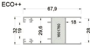
360-1301* ( 1,820 kg/mt ) ÜÇ RAYLI KASA PROFİLİ
