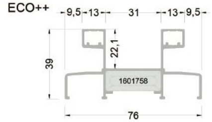
360-1211 ( 0,858 kg/mt ) 2 RAYLI KASA PROFİLİ
