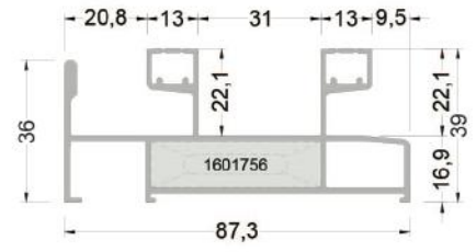
360-1205 ( 1,360 kg/mt ) SİNEKLİK RAYLI İKİLİ KASA PROFİLİ
