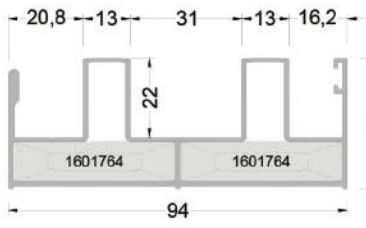
360-1207 ( 1,245 kg/mt ) SİNEKLİK RAYLI ÜST/YAN KASA PROFİLİ
