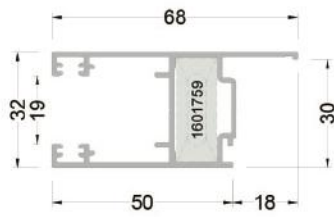
360-2102 ( 0,820 kg/mt ) KANAT PROFİLİ
