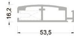
380-4003 ( 0,661 kg/mt ) S72S03 SİNEKLİK KANAT PR.
