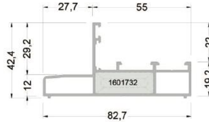
360-3101* ( 0,972 kg/mt ) SABİT GEÇİŞ KASA PROFİLİ
