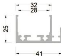
360-6002 ( 0,610 kg/mt ) MİNİMAL KENET PROFİLİ
