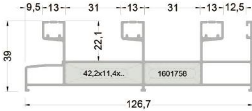
360-1301* ( 1,820 kg/mt ) ÜÇ RAYLI KASA PROFİLİ
