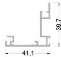
360-6001 ( 0,433 kg/mt ) KENET PROFİLİ
