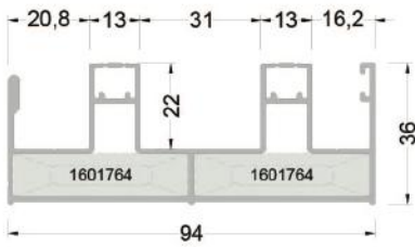
360-1206 ( 1,330 kg/mt ) SİNEKLİK RAYLI ALT KASA PROFİLİ
