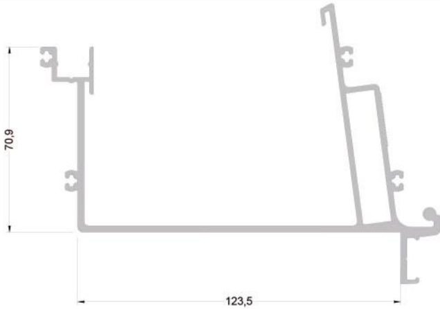
560-6104 ( 0,785 kg/mt ) ADAPTÖR PROFİLİ
