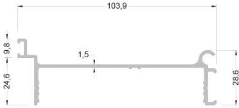
560-6104 ( 0,785 kg/mt ) ADAPTÖR PROFİLİ
