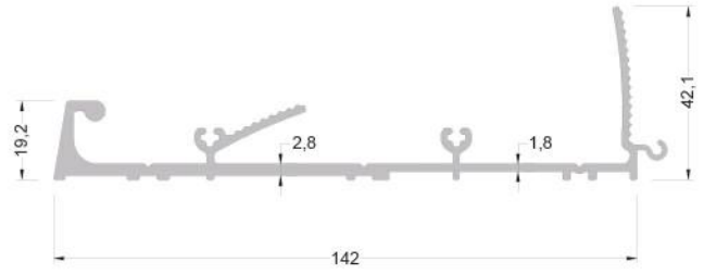
560-6201 ( 1,722 kg/mt ) DUVAR BAĞLANTI PROFİLİ
