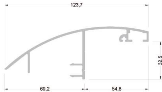
560-6106 ( 0,579 kg/mt ) ADAPTÖR PROFİLİ
