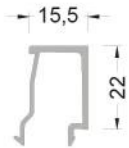
800-155 ( 0,249 kg/mt ) G155 CAM ÇİTASI
