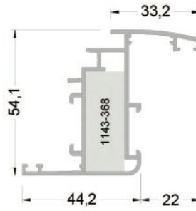
145-3101 ( 0,951 kg/mt ) WA45V01 DAR KANAT PROFİLİ
