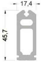
1143 ( 2,867 kg/mt ) L143 KÖŞE TAKOZU
