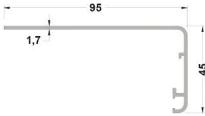
801-140 ( 0,605 kg/mt ) AW14 PERVAZ PROFİLİ
