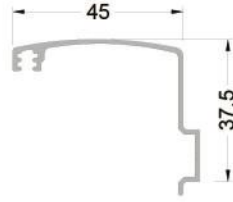
801-410 ( 0,343 kg/mt ) AW03 PERVAZ PROFİLİ
