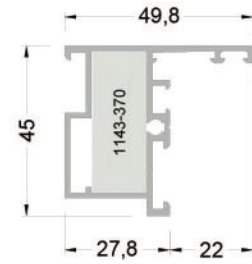
145-5102 ( 0,771 kg/mt ) WA45A02 DIŞ AÇILIM KANAT ADAPTÖR PROFİLİ
