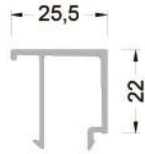
803-101 ( 0,186 kg/mt ) P01 DAMLALIK PROFİLİ
