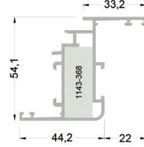
145-3102 ( 0,940 kg/mt ) WA45V05 DAR KANAT PROFİLİ
