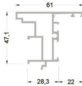
145-5101 ( 1,011 kg/mt ) WA45A01 ÇİFT KANAT ADAPTÖR PROFİLİ
