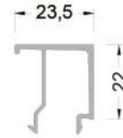
803-101 ( 0,186 kg/mt ) P01 DAMLALIK PROFİLİ
