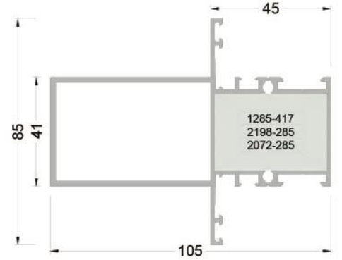
145-2501 ( 1,918 kg/mt ) WA45M04 TAKVİYELİ ORTA KAYIT PROFİLİ
