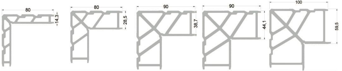
1143 ( 2,867 kg/mt ) L143 KÖŞE TAKOZU
