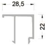
804-101 ( 0,110 kg/mt ) IW01 TİJ PROFİLİ
