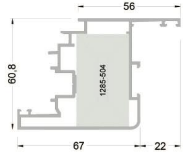
145-3602 ( 1,351 kg/mt ) WA45V08 PVC KANAT PROFİLİ
