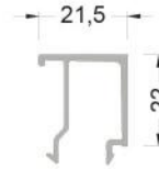
801-135 ( 0,357 kg/mt ) AW12 PERVAZ PROFİLİ
