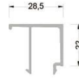
800-285 ( 0,300 kg/mt ) G285 CAM ÇİTASI
