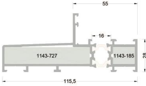
320-1404 (1,926 kg/mt.) ST120F09 SABİT GEÇİŞ KASA PROFİLİ
