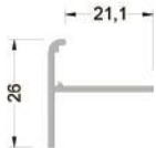
802-101 ( 0,185 kg/mt ) T01 T BİNİ PROFİLİ
