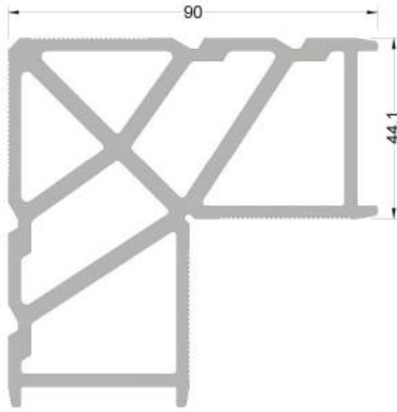
1441 ( 5,116 kg/mt ) L441 KÖŞE TAKOZU
