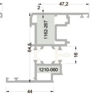
255-3608 ( 1,736 kg/mt ) T55V27 PVC KANAT PR.
