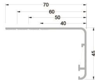
801-070 ( 0,525 kg/mt ) AW13 PERVAZ PROFİLİ
