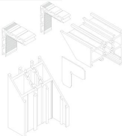
1441 ( 5,116 kg/mt ) L441 KÖŞE TAKOZU
