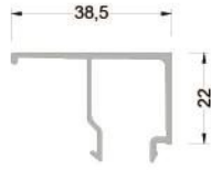
800-385 ( 0,332 kg/mt ) G385 CAM ÇİTASI
