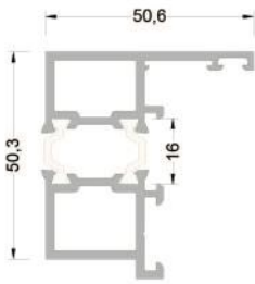
T55A08* ( 1,492 kg/mt ) 90° DÖNÜŞ ADAPTÖR PR.
