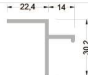
802-104 ( 0,126 kg/mt ) T-4680 T BİNİ PROFİLİ
