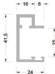
255-5205 ( 0,610 kg/mt ) T55 A06 EŞİK PROFİLİ
