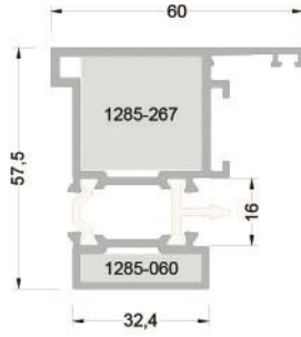
255-5104 ( 1,492kg/mt ) T55A04 PİVOT ADAPTÖR PR.
