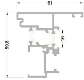
255-5102 ( 1,358 kg/mt ) T55A02 ÇİFT KANAT ADPTR PR.
