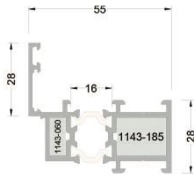
255-5104 ( 1,492kg/mt ) T55A04 PİVOT ADAPTÖR PR.
