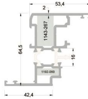
255-3604 ( 1,750 kg/mt ) T55V17 PVC KANAT PR.
