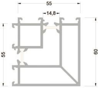
T55A08* ( 1,492 kg/mt ) 90° DÖNÜŞ ADAPTÖR PR.
