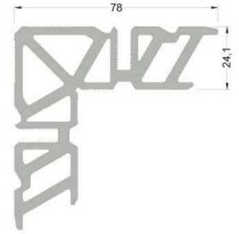
1241 ( 3,799 kg/mt ) L241 KÖŞE TAKOZU
