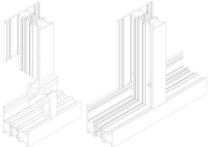
2198 ( 1,170 kg/mt ) ORTA KAYIT BAĞLANTI PROFİLİ
