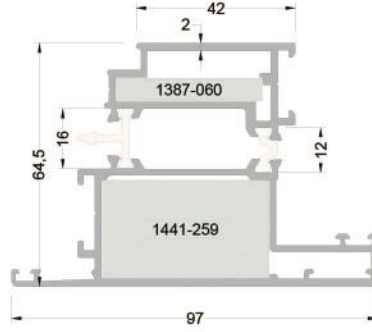
255-3403 ( 2,329 kg/mt ) T55V11 DIŞ AÇILIM KAPI KANAT PR.
