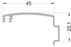
801-288 ( 0,377 kg/mt ) AW02 PERVAZ PROFİLİ
