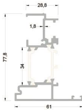
273-5102 ( 1,419 kg/mt ) WAT73A02 PVC KANAT ADP.PR.
