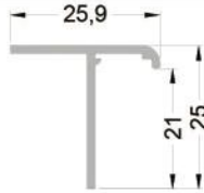
802-101 ( 0,185 kg/mt ) T01 T BİNİ PROFİLİ
