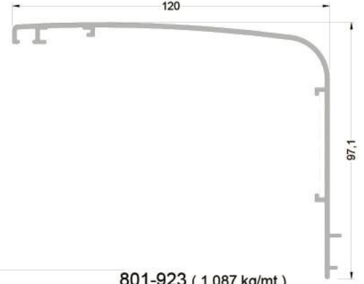
801-923 ( 1,087 kg/mt ) AW10 PERVAZ PROFİLİ
