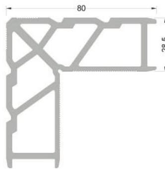
1162 ( 2,783 kg/mt ) L162 KÖŞE TAKOZU
