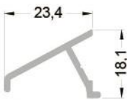
803-101 ( 0,186 kg/mt ) P01 DAMLALIK PROFİLİ
