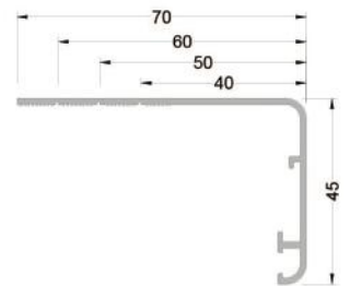
801-070 ( 0,525 kg/mt ) AW13 PERVAZ PROFİLİ
