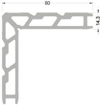
1143 ( 2,867 kg/mt ) L143 KÖŞE TAKOZU
