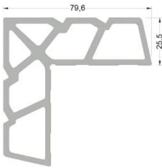
1143 ( 2,867 kg/mt ) L143 KÖŞE TAKOZU
