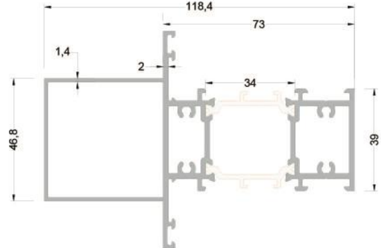
273-2502 (2,498 kg/mt) WAT73 TAKVİYELİ ORTA KAYIT PROFİLİ
