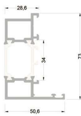
273-5103 ( 1,409 kg/mt ) WAT73A03 DIŞ AÇILIM ADP. PR.
