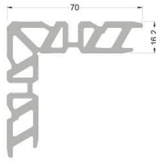
1162 ( 2,783 kg/mt ) L162 KÖŞE TAKOZU
