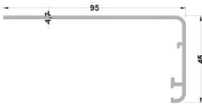
801-140 ( 0,605 kg/mt ) AW14 PERVAZ PROFİLİ
