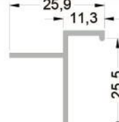
802-102 ( 0,188 kg/mt ) T02 T BİNİ PROFİLİ
