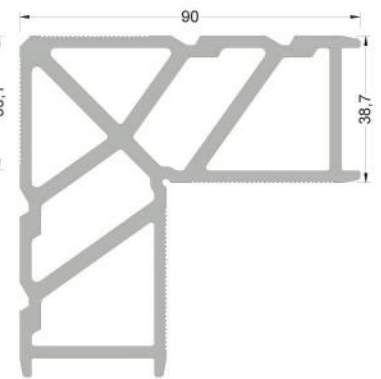
1387 ( 4,924 kg/mt ) L387 KÖŞE TAKOZU
