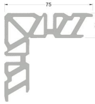
1210 ( 3,449 kg/mt ) L210 KÖŞE TAKOZU
