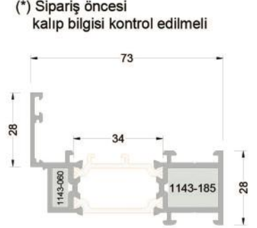
273-5105* ( 1,517 kg/mt ) T73A05 KANAT İÇİ KANAT ADP.
