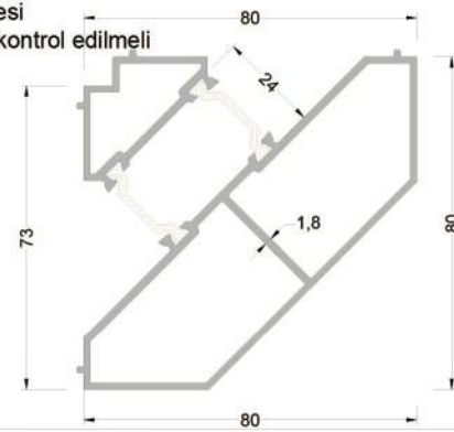
273-5106* ( 1,970 kg/mt ) T73A06 90° DÖNÜŞ ADAPTÖR PROFİLİ
