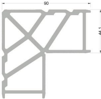
1441 ( 5,116 kg/mt ) L441 KÖŞE TAKOZU
