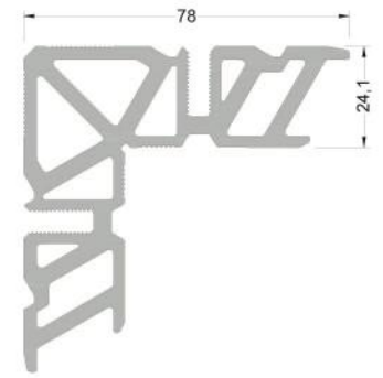
1241 ( 3,799 kg/mt ) L241 KÖŞE TAKOZU
