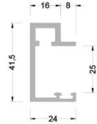
AS-8255 ( 0,681 kg/mt ) CAM KORKULUK DİKME PR.
