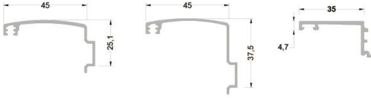
801-288 ( 0,377 kg/mt ) AW02 PERVAZ PROFİLİ
