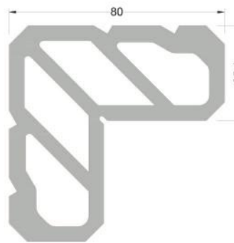
1210 ( 3,449 kg/mt ) L210 KÖŞE TAKOZU
