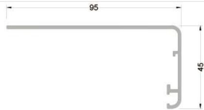
801-140 ( 0,6005 kg/mt ) PERVAZ PROFİLİ
