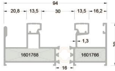
370-1202* ( 1,620 kg/mt ) SİNEKLİK RAYLI KASA PROFİLİ
