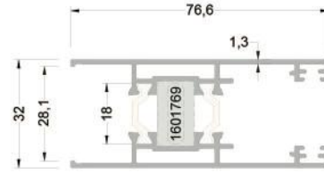
370-1203* ( 1,602 kg/mt ) SİNEKLİK RAYLI KASA PROFİLİ
