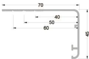
801-070 ( 0,522 kg/mt ) PERVAZ PROFİLİ
