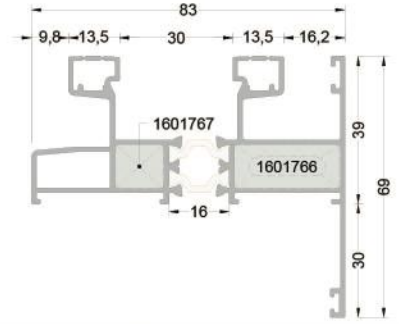
370-1203* ( 1,602 kg/mt ) SİNEKLİK RAYLI KASA PROFİLİ
