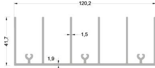
350-1103 ( 1,783 kg/mt ) SSA120 ÜST KASA PROFİLİ 120MM
