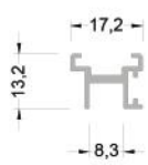
350-6101* (0,159 kg/mt ) SSA120 ÜST ADP. PR. 8 MM 350-6103 (0,173 kg/mt ) SSA120 ÜST ADP. PR. 10 MM 350-6102* (0,098 kg/mt ) SSA120 KENET ADP. PR. 8 MM 350-6106 (0,189 kg/mt ) SSA120 KENET ADP. PR. 10 MM 350-6105 (0,175 kg/mt ) SSA120 ÜST ADP. PR. 10 MM
