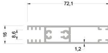
350-2102* (0,866 kg/mt ) SSA120 KANAT PROFİLİ 8MM
