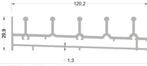
350-1101 ( 1,837kg/mt ) SSA120 EŞİKLİ KASA PROFİLİ 5'Lİ
