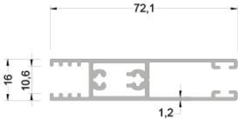
350-2101 (0,840kg/mt ) SSA120 KANAT PROFİLİ 10MM
