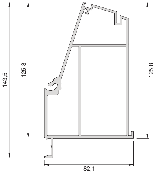
580-2101 ( 3,438 kg/mt ) SRA150 T01 ŞAŞİ PROFİLİ
