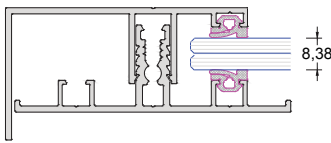
4.4 Lamine Cam 0,38 PvP
