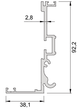
580-5102 ( 1,373 kg/mt ) SRA150 A10 AÇI İLETİM PROFİLİ
