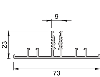
580-2101 ( 3,438 kg/mt ) SRA150 T01 ŞAŞİ PROFİLİ
