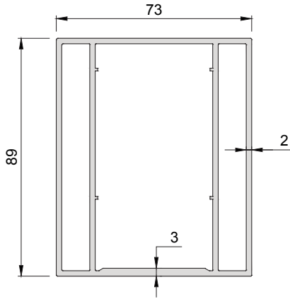
580-1201 ( 2,743 kg/mt ) SRA150 M03 TAŞIYICI DİKME PROFİLİ
