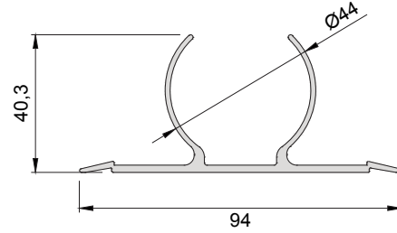
580-5101 ( 0,879 kg/mt ) SRA150 A09 BAĞLANTI PROFİLİ
