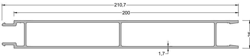
700-3105 ( 2,359 kg/mt ) ÇİT PANEL PROFİLİ
