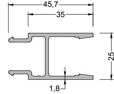
700-3101 ( 0,243 kg/mt ) GFA100 SEKİZGEN ÇİT PR.
