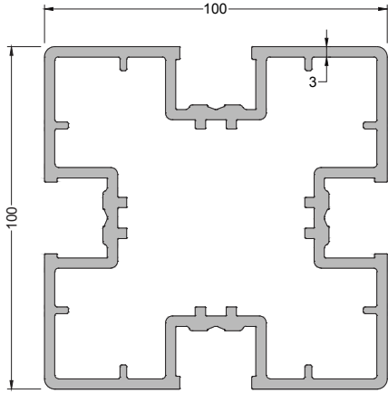
700-1101 ( 4,985 kg/mt ) GFA100 ÇİT DİKME PROFİLİ
