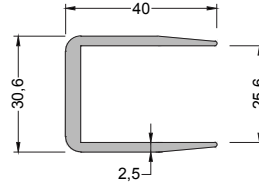
700-2102 ( 0,743 kg/mt ) ÇİT U PROFİLİ
