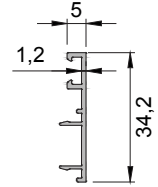
645-7201 ( 0,174 kg/mt ) IPA45P04 KAPAK PROFİLİ
