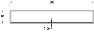
700-3102 ( 0,827 kg/mt ) GFA100 ÇİT KUTU PROFİLİ
